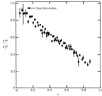
Abbildung 1: Messung von F_2^{en}/F_2^{ep} als Funktion von x in tiefinelastischer Streuung.
